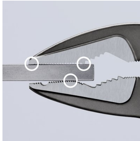
Lange, spitze Backen mit Frontgreif-Verzahnung: längs eingebrachtes Greifprofil für Rundteile wie Schrauben und Bolzen sicherer Griff auch an Flachteilen durch Dreipunktauflage
