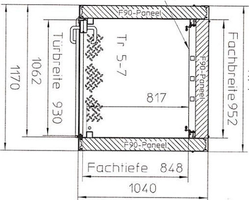
Schnitt A-A 1171
