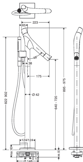
完成図
