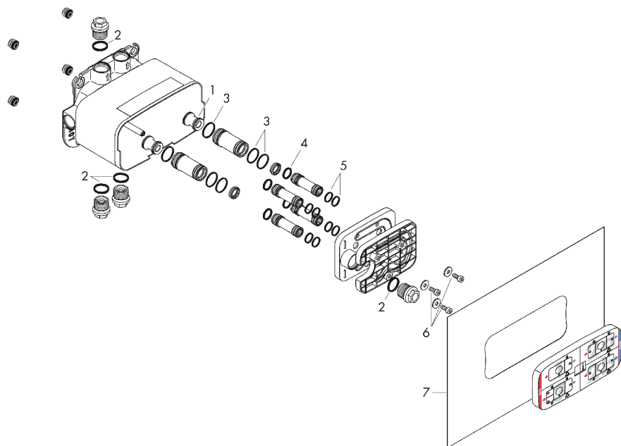
製品分解図
