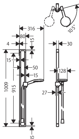
完成図
