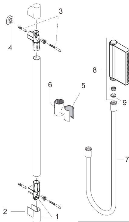
製品分解図
