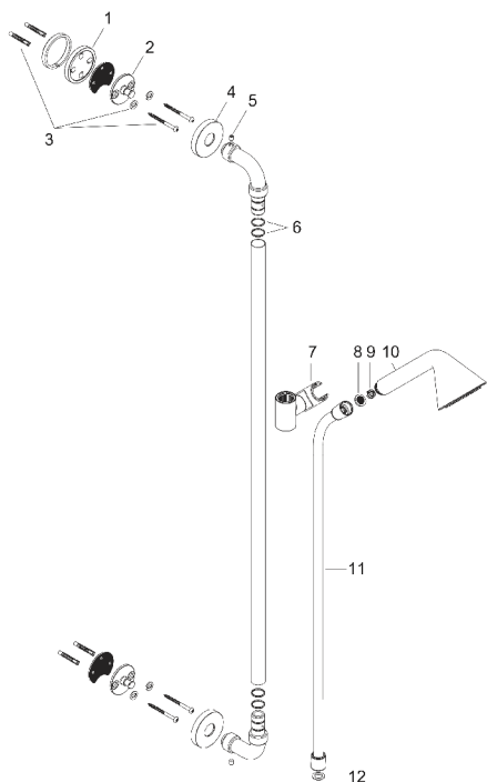
製品分解図
