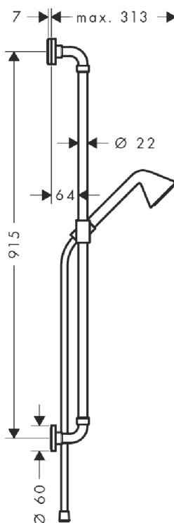
完成図
