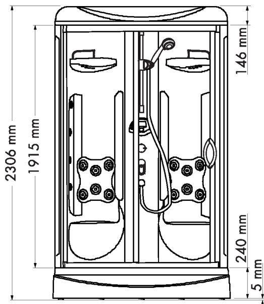
Vue intérieure Vista interior Indvendig tegning
