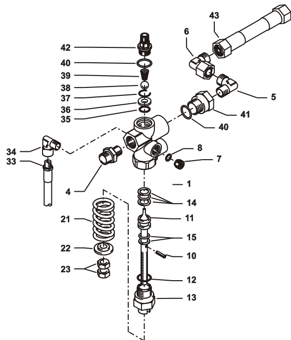
Veiligheidsventiel voor verwarmingsspiraal (Instelling moet ca. 15% hoger als de bedrijfsdruk zijn)
