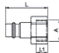
Nippel Innengewinde
