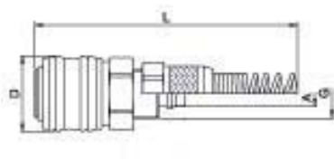
Schlauchanschluss, Überwurfmutter und Knickschutzfeder
