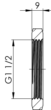
SCHNITT A-A
