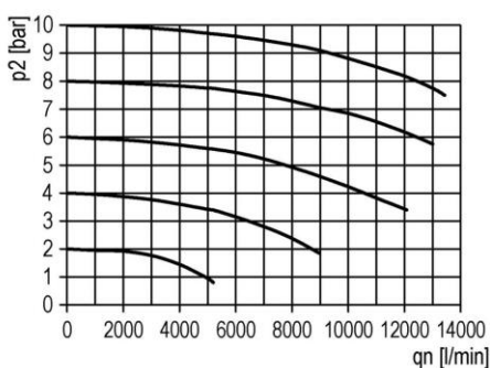
Durchflussdiagramm
