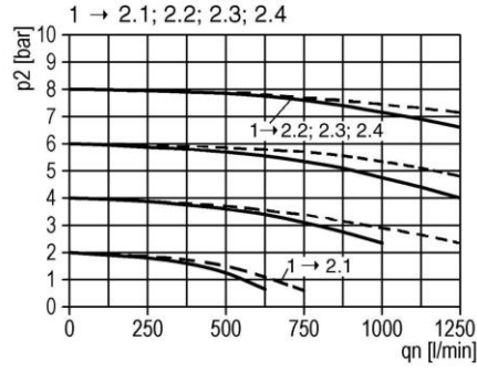
2. Durchflussdiagramm
