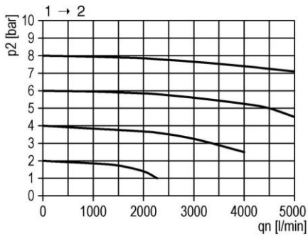
1. Durchflussdiagramm
