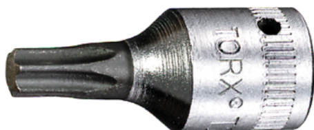
01350030 44 KTX T 30 SCHRAUBENDREHEREINSATZ 1/4 ZOLL 6,3 mm (1/4") Schraubendrehereinsatz TORX T30 L.28 mm
