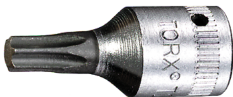
01350027 44 KTX T 27 SCHRAUBENDREHEREINSATZ 1/4 ZOLL 6,3 mm (1/4") Schraubendrehereinsatz TORX T27 L.28 mm
