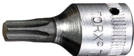
01350008 44 KTX T 8 SCHRAUBENDREHEREINSATZ 1/4 ZOLL 6,3 mm (1/4") Schraubendrehereinsatz TORX T8 L.28 mm
