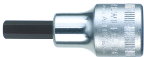
03050007 54 7 12,5 mm (1/2") INHEX-Einsatz 7 mm L.60 mm
