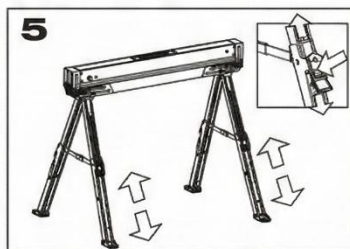
Le gambe possono essere regolate a passi di 2,54 cm. Per allungare, tirare giù le gambe fino a quando il chiavistello non si trova nella posizione desiderata. Per ritirare, premere il pulsante di bloccaggio, spingere leggermente verso il basso e successivamente spingere su la gamba.
