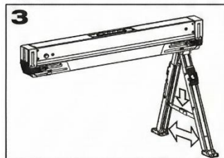
Speizen Sie die Beine und drücken Sie die Querstange nach unten.
