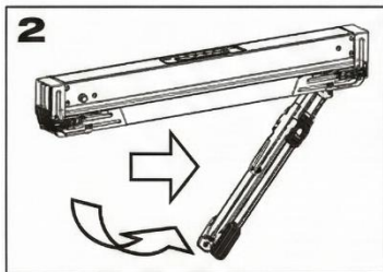
Nad oznaczeniem "OTWÓRZ NAJPIERW", naciśnij przycisk zwalnający i pociągnij nogę w dół, aż zostaną w pełni rozłożone.
