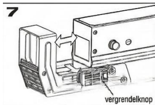
Spreid de poten en duw de dwarsbalk omlaag.
