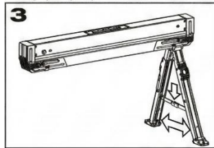
Spreid de poten en duw de dwarsbalk omlaag.
