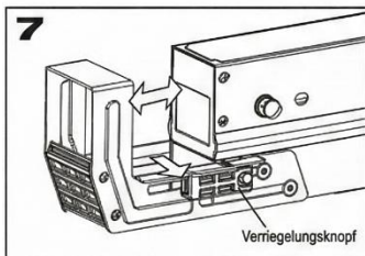
Öffnen Sie den Verriegelungsknopf und passen Sie die Seitenhalterung auf die gewünschte Breite an. Ziehen Sie den Knopf fest, sobald der Balken eingesetzt ist. Einstellbar zwischen 0 mm und 90 mm für verschiedene Balken.
