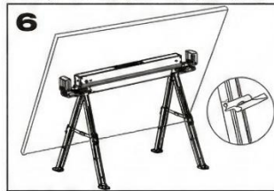
Klap de steunpennen uit om een plaat te ondersteunen voor het zagen.
