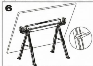
Klappen Sie die Haltestifte aus, um eine Platte zum Schneiden zu stützen.
