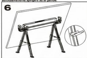
Spiegare i perni di supporto per sostenere una piastra per il taglio.
