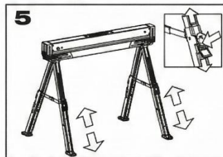
Die Beine können in Stufen von 2,54 cm verstellt werden. Zum Ausfahren ziehen Sie die Beine nach unten, bis der Riegel in der gewünschten Position einrastet. Zum Einfahren drücken Sie den Sperrknopf, ziehen Sie das Bein leicht nach unten und drücken Sie es
