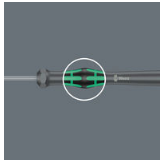
Die Kraftzone mit integrierten Weichzonen in Nähe der Klingenspitze sorgt für die Übertragung hoher Löse- und Anzugsmomente, ohne dass der Kontakt zur Schraube verloren geht.
